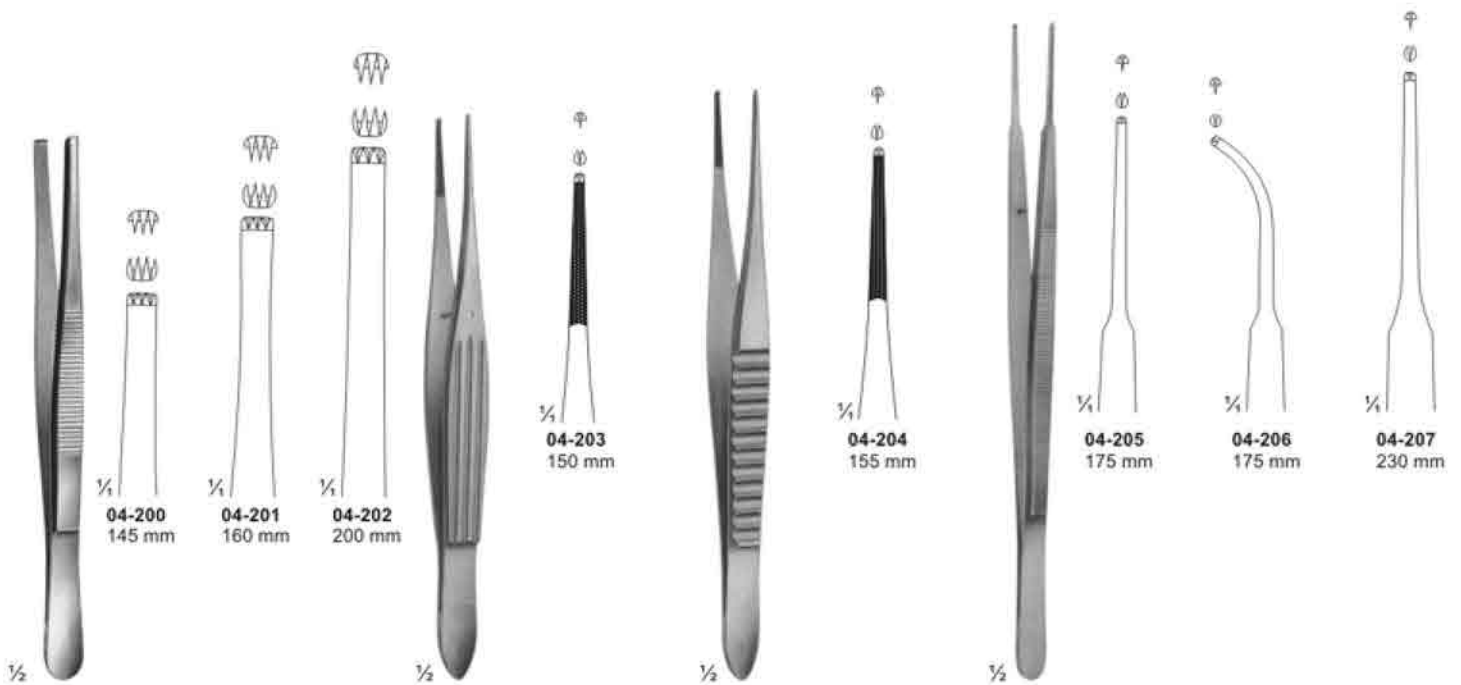
04-200 - 04-203 3x4 teeth
